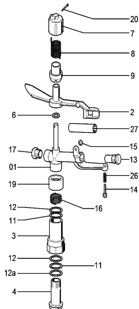
ZENITH TESO 6° cod. 10249
